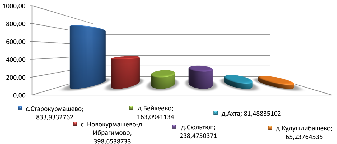
Рис: Расход газа по населенным пунктам в перспективе до 2033 г.
